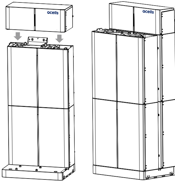
Vier Batteriemodule
