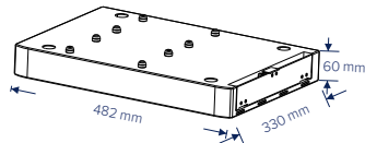
Doppel-Batteriesockel
