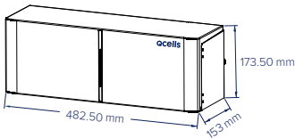
BMS (Q.SAVE BMS-G3)
