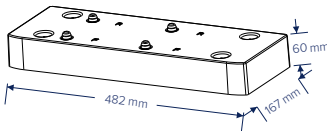
Einzel-Batteriesockel
